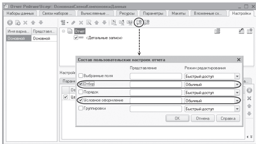
Рис. 13.49. Состав пользовательских настроек
